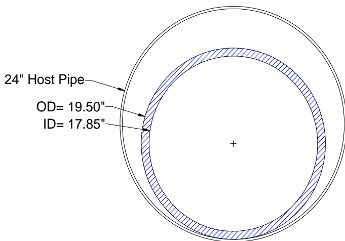
18" DR 25 Fusible C-905®
